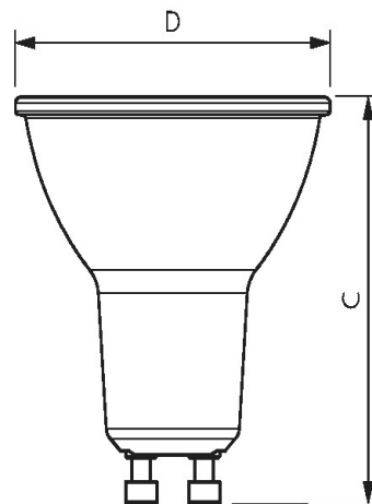
Abmessungsskizze
